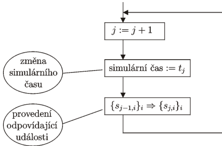
Obrázek 3.1: Schéma základního cyklu simulačního programu [33]
